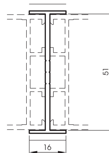
5022 Liaison section 50
