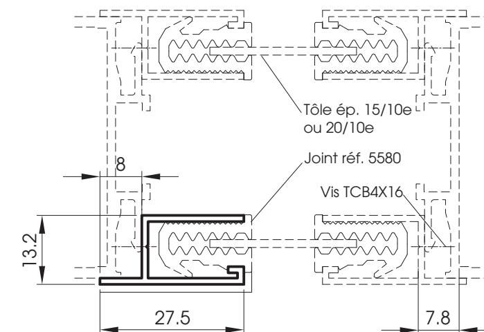
5138 Profil de dilatation
