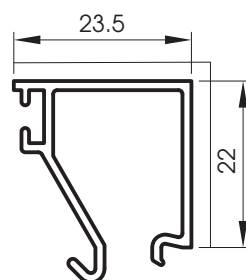
5054 Parclose clipable 23.5 mm
