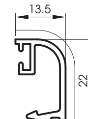
5512 Parclose arrondie 13.5 mm
