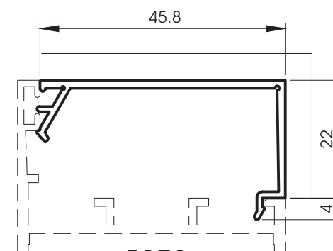
5978 Closir de feuillure gamme 5000/50
