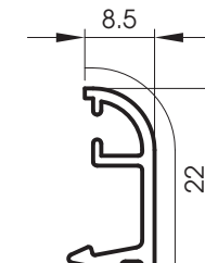
5511 Parclose arrondie 8.5 mm
