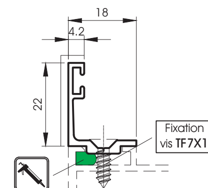
5049 Parclose à visser
