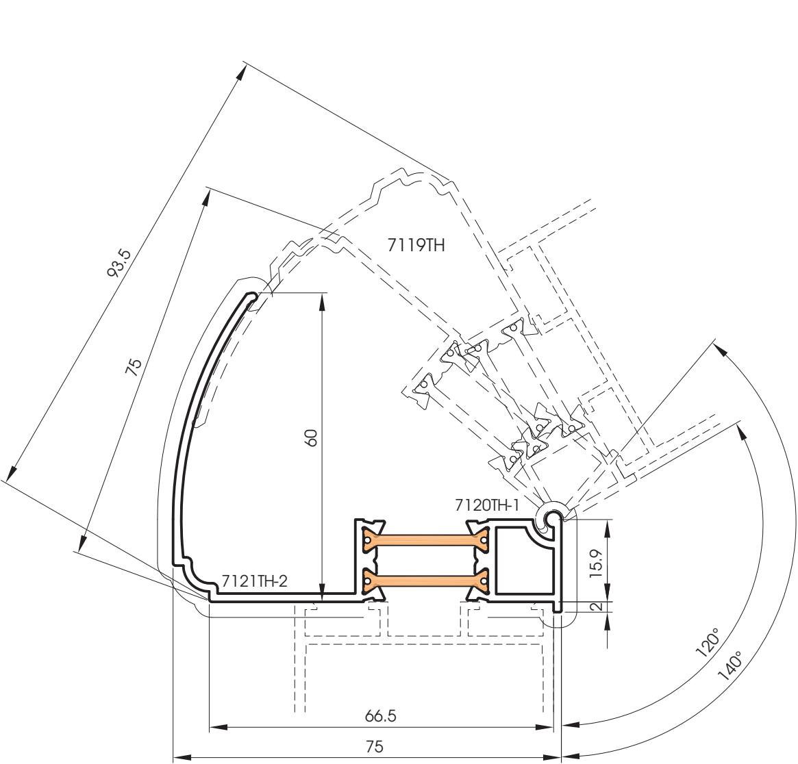
7121TH Poteau variable pour angle de 120° à 140°
