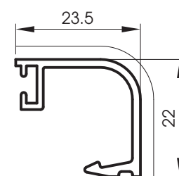
5514 Parclose arrondie 23.5 mm
