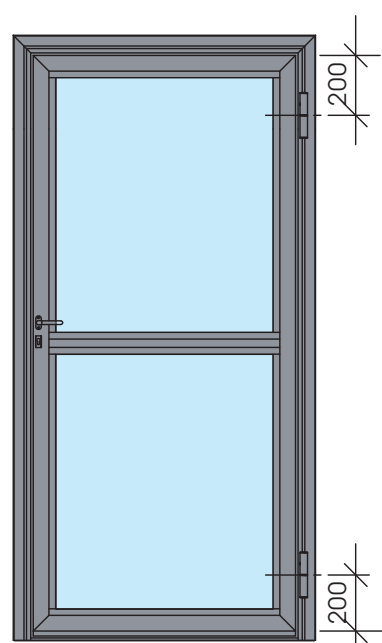
2 PAUMELLES
