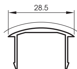
5057 Capot profil 5041-5042
