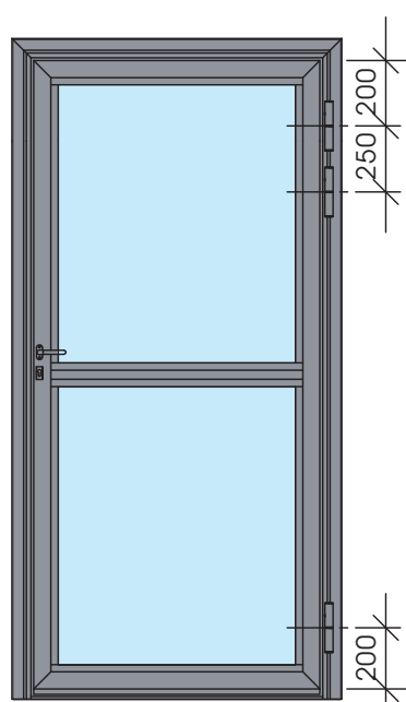
3 PAUMELLES
