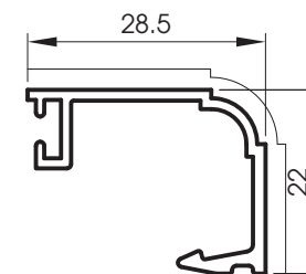
5521 Parclose moulurée 28.5 mm
