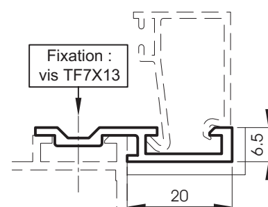
5058 Élargisseur de feuillure
