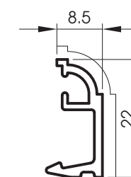
5517 Parclose moulurée 8.5 mm
