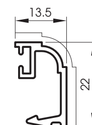
5518 Parclose moulurée 13.5 mm
