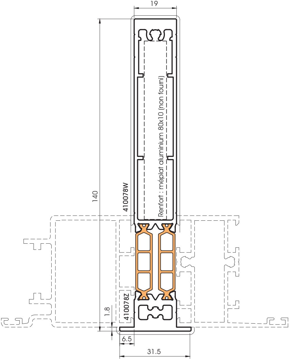
410078 Renfort 50-70
