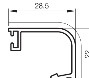
5515 Parclose arrondie 28.5 mm
