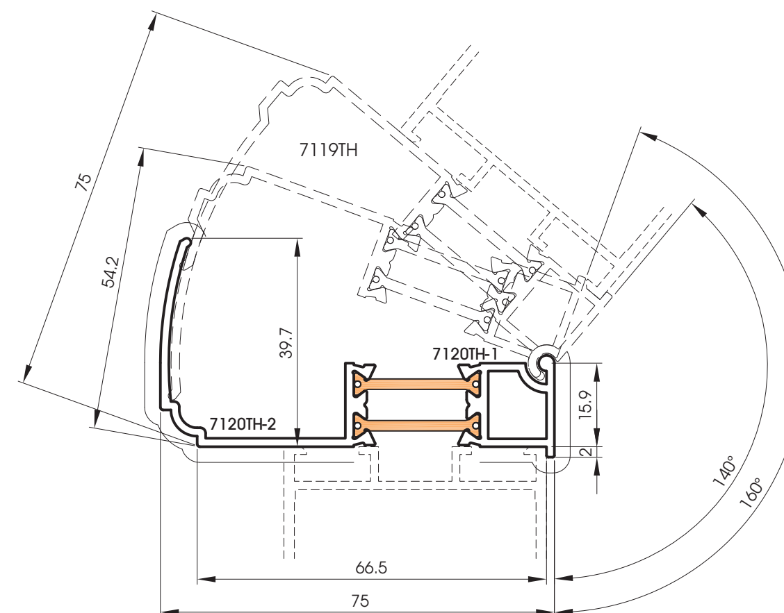
7120TH Poteau variable pour angle de 140° à 160°
