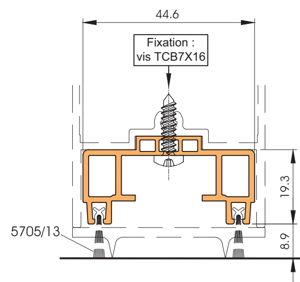
P5063 Profil porte-joint
