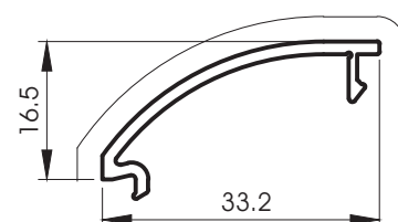
P5058 Finition haute P5055
