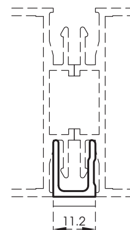
6598/4 Liaison couvre-joint lg. 4600 mm
